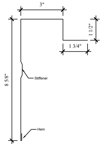
20RT Door Top
