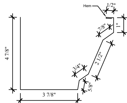
6" K-Gutter No Flange
