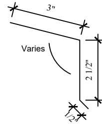
Gutter Apron
