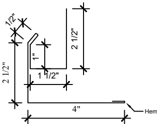
19R Sliding Door Facer
